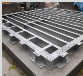
架台設置
